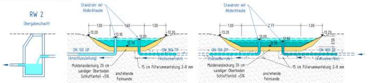
Längsschnitt Versickerungsanlage (schematisch) M 1:50
